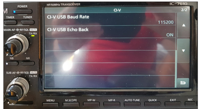
Konfiguration der Übertragungsrate der CI-V-Schnittstelle im Icom IC-7610
