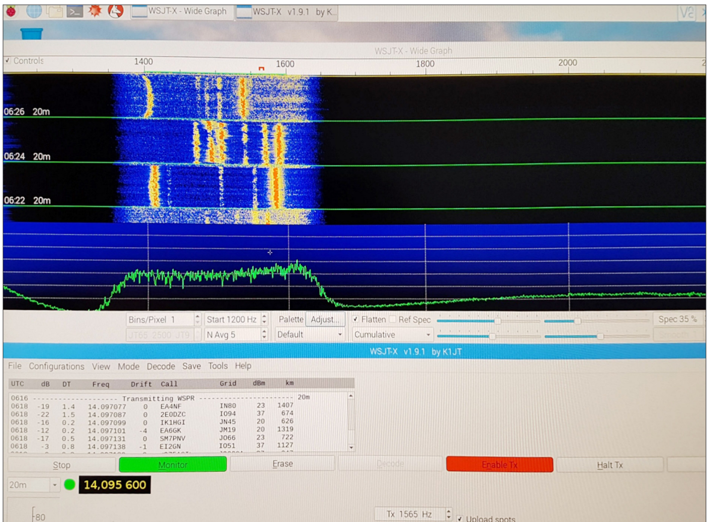
Einstellung des Programms WSJT-X zur korrekten Darstellung des Wasserfalldiagramms
