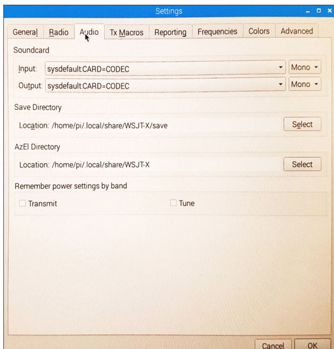
Einstellungen für die Audio-Verbindung mit dem Icom IC-7610 im Programm WSJT-X
