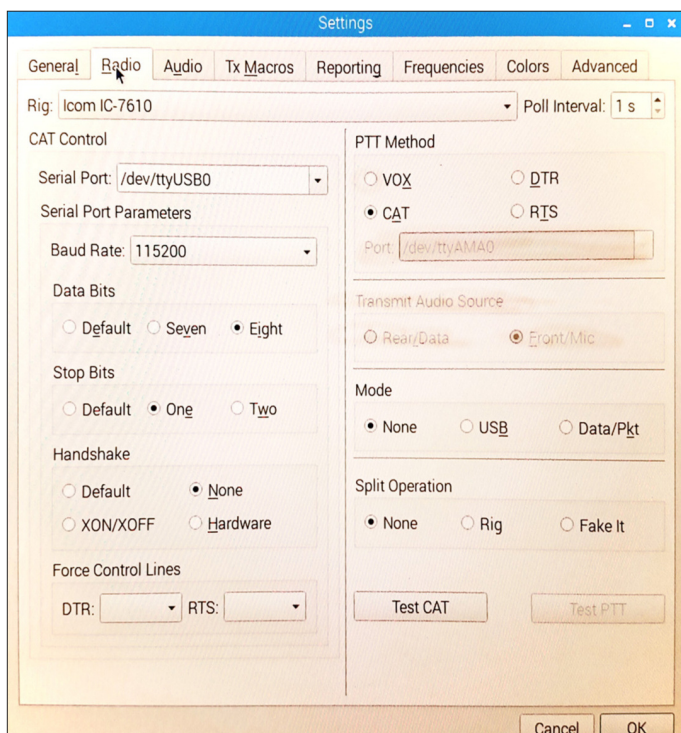
Einstellungen für die Kommunikation mit dem Icom IC-7610 im Programm WSJT-X
